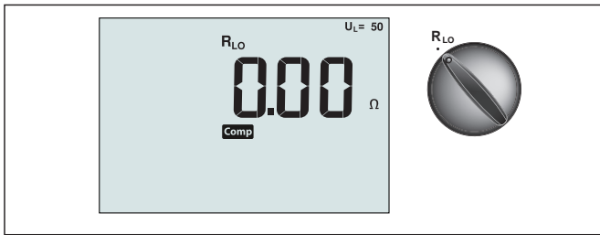
Figur 10. Visning og bryter-/kontaktinnstillinger for kontinuitet null
