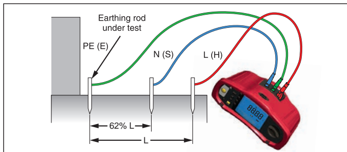
Fig. 20. Tilslutning for test af jordmodstand
