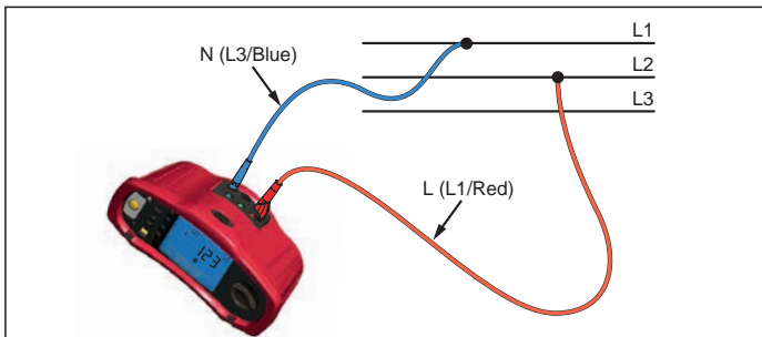
Abbildung 15. Messung in einem Dreiphasensystem
