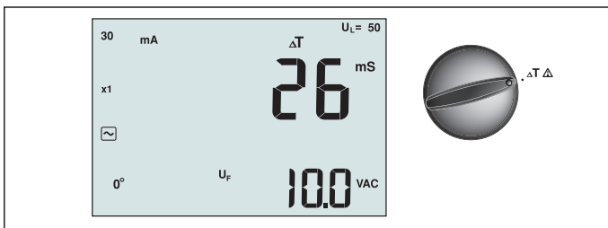
Afbeelding 16. Weergave RCD triptijd/Instellingen schakelaar en aansluitingen
