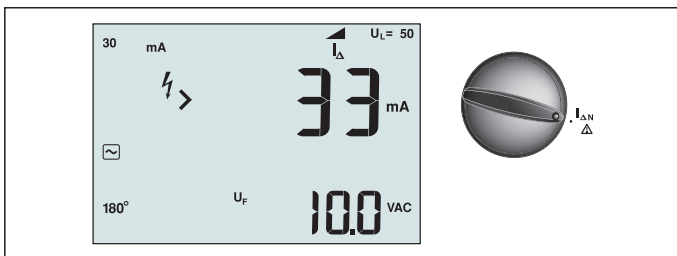
Afbeelding 17. RCD tripstroom/Instellingen schakelaar en aansluitingen
