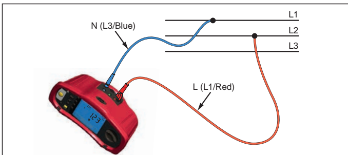
Figur 15. Mätning i ett 3-fasystem
