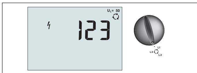
Figur 21. Visning av fäsföljd/Inställningar för växling och poler
