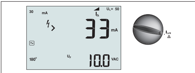
Kuva 17. Vikavirtasuojien laukaisuvirran näyttö / Kytkin- ja liitinasetukset
