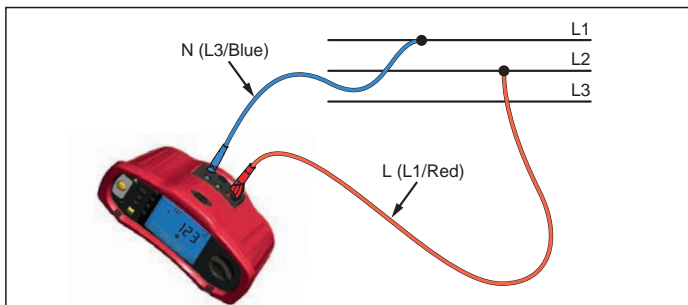
Fig. 15. Måling i et 3-fase system
