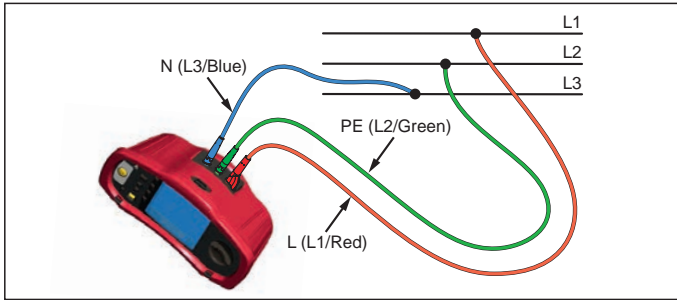
Kuva 22. Vaihejärjestystestin kytkenä
