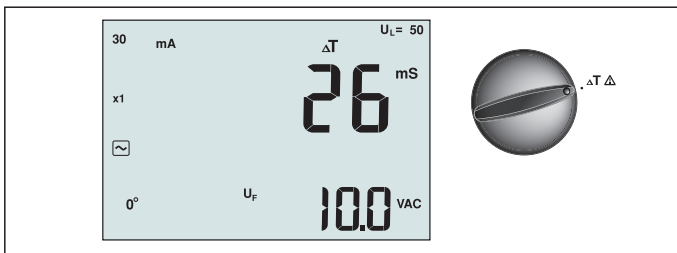
Figur 16. Visning av RCD-utlösningstid/Inställningar för växling och poler
