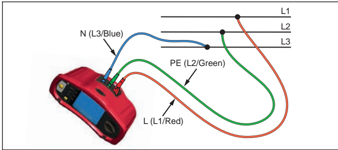
Figur 22. Fasesekvenstesttilkobling
