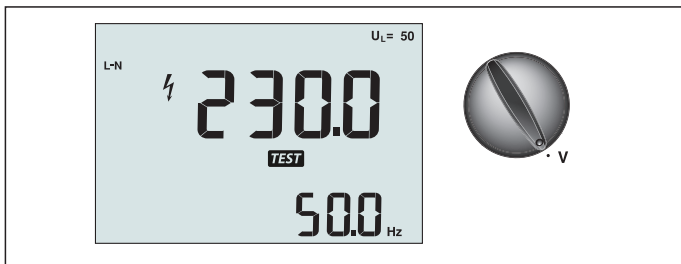
Rysunek 8. Wyświetlacz/Przełącznik voltów i ustawienia złącza
