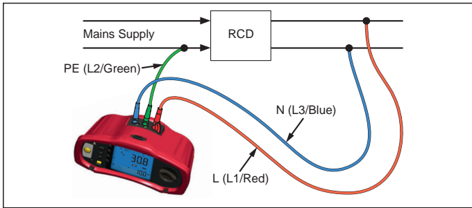
Rysunek 18. Podłączenie przy testowaniu wyłączników RCD w systemach elektrycznych IT Prąd testowy płynie przez górną część wyłącznika RCD do złącza L, i powraca poprzez złącze PE.
