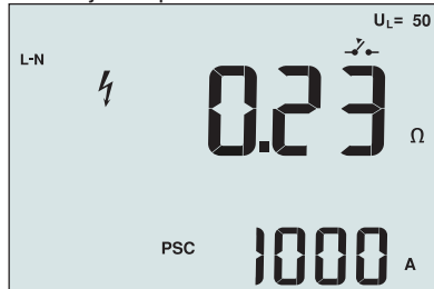
Kuva 14. Linjaimpedanssin näyttö
