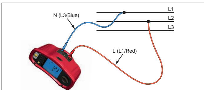
Rysunek 15. Pomiar w systemie trójfazowym
