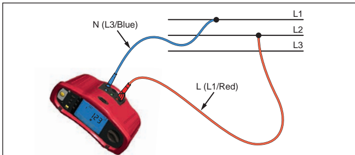
Kuva 15. Mittaus kolmivaihejärjestelmässä
