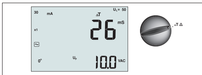
Rysunek 16. Wyświetlacz czasu wyzwiania RCD/Ustawienia przełącznika oraz złącza
